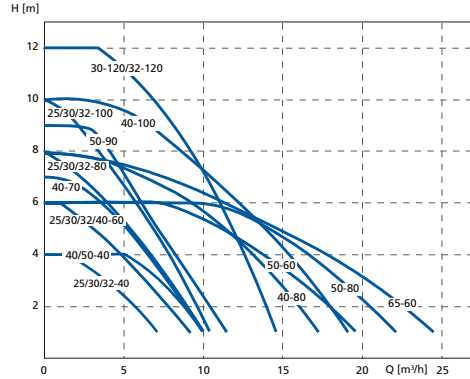
Calio Pro Karakteristik Eğriler
