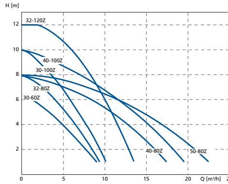
Calio Pro Z Karakteristik Eğriler
